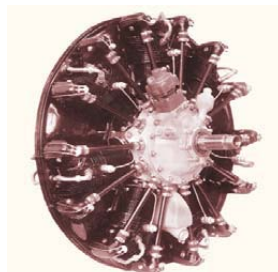
Двигатель АИ-14Р
